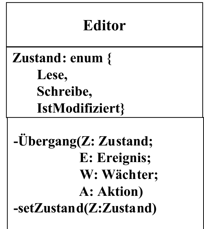
Zugehöriges Klassendiagramm
