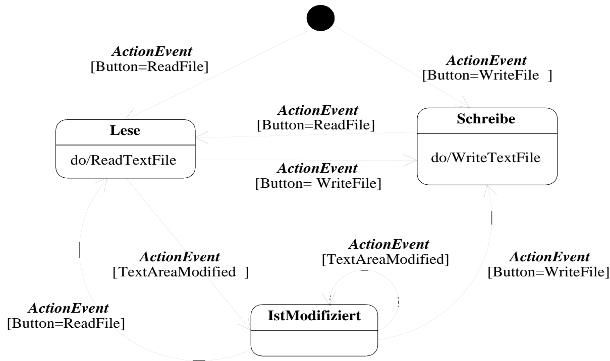
Zustandsdiagramm
